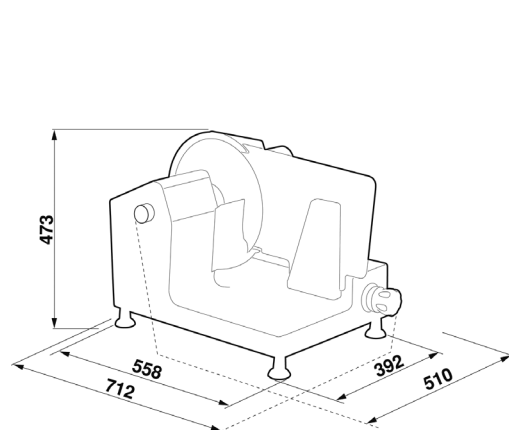
Dimensions Gravinox 300V
